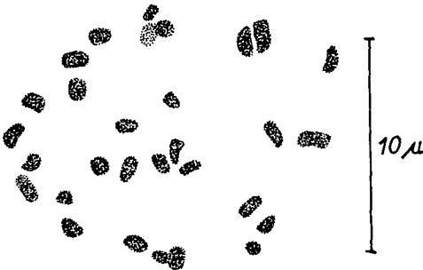
Abb. 2. Lasius (Chthonolasius) flavus . 2n=30 . Oogonienmitose.
