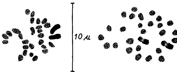
Abb. 6. Lasius (Lasius) alienus . 2n = 28 . Neuroblastenmitose.
