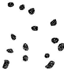
Abb. 9. Strongylognathus huberi alpina . n = 14 . Spermatogonienmitose.
