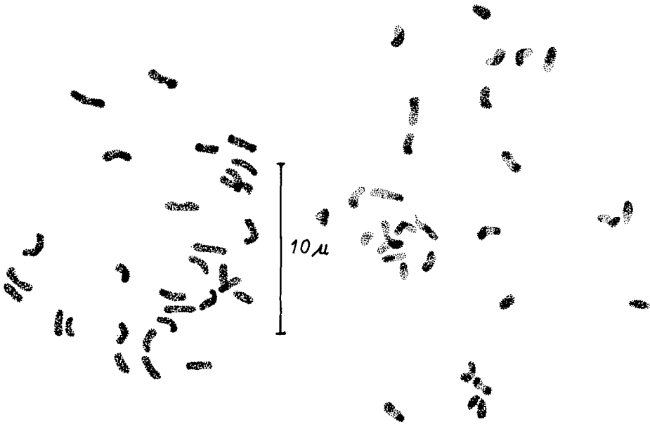
Abb. 4. Lasius (Lasius) niger . 2n = 30 . Oogonienmitose.
