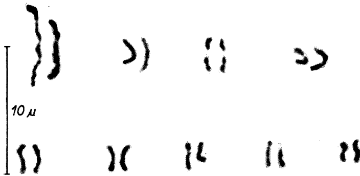
Abb. 13. Leptothorax tuberum tuberum . Karyotyp einer Neuroblastenmitose.
