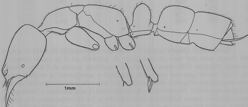
Fig. 3. Belonopelta attenuata MAYR, profilo schematico dell'operaia lectotipica.
