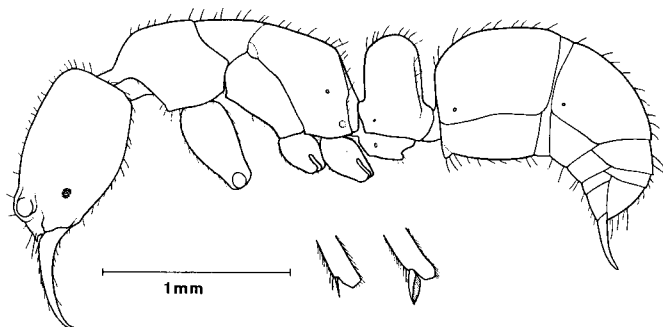
Fig. 5. Belonopelta buttelreepeni (FOREL), profilo schematico dell'olotipo operaia.
