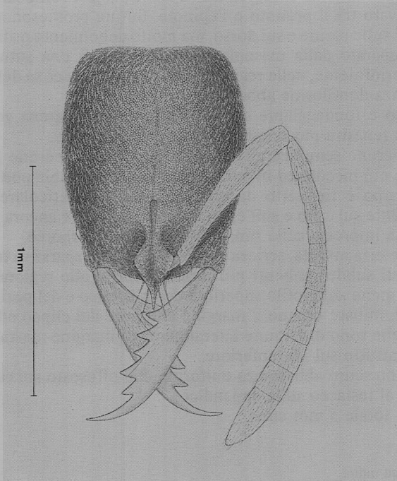
Fig. 2. Belonopelta attenuata MAYR, capo dell'operaia paralectotipica in visione dorsale.
