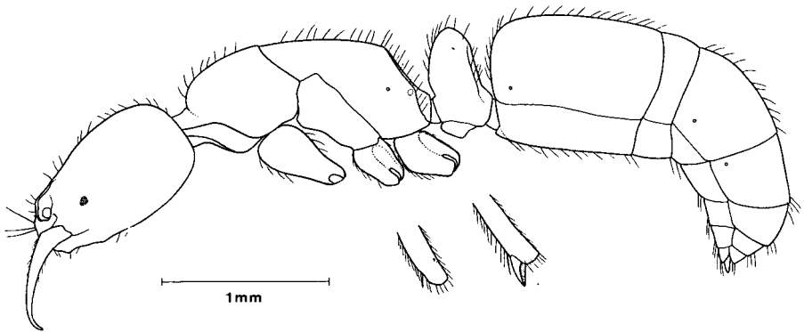
Fig. 6. Belonopelta franzi n.sp., profilo schematico dell'operaia olotipo.
